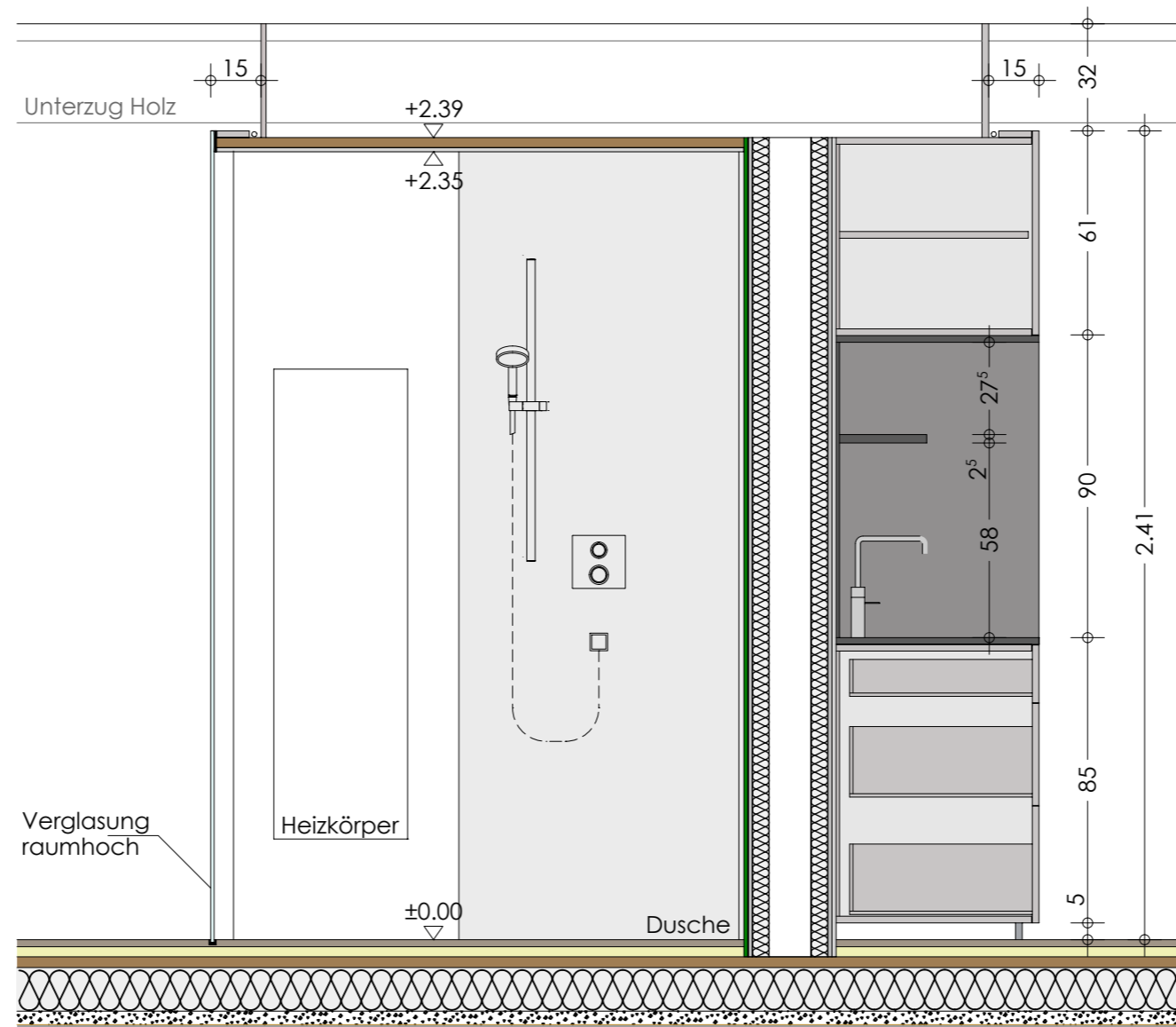
Schnitt 7-7 M 1:20
